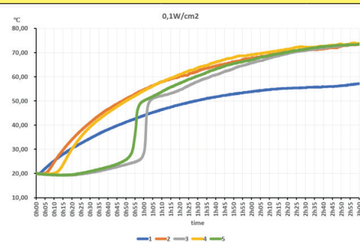
Bei einer Oberflächenlast von 0,1 W/cm 2 (60 W)
