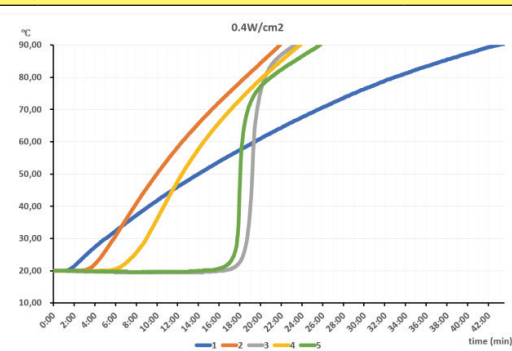
Bei einer Oberflächenlast von 0,4W/cm 2 (240W)
