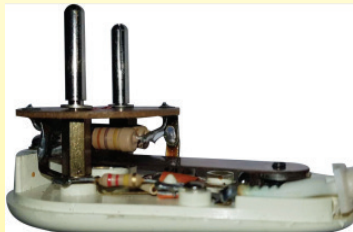
Ca. 1972. Schaltkasten der Firma Jidé in Limoges unter der Marke Jidéstat. Das erfolgreichste aller Systeme. Es ist sehr klein, einstellbar und in den Stecker integriert. Dies ist das einzige Modell mit einem Schnappmagnetkontakt. Es wurde erst in der heutigen Zeit von elektromechanischen Systemen überholt. (Ultimheat-Sammlung)
